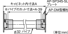
パイプソケット抜け止め
